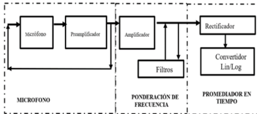
FIGURA 1. Esquema sonómetro. Autores
