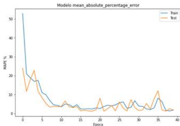
FIGURA 8. Tendencia MAPE Elaboración Propia
