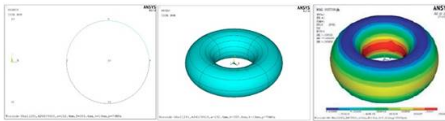
FIGURA 1. Toroide de Sección Recta Circular (Patiño & Corz, 2018)
