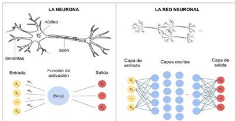
FIGURA 2. La Neurona y la Red Neuronal Artificial Propia
