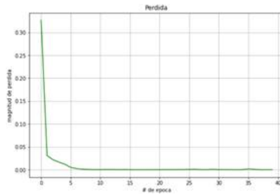
FIGURA 10. Tendencia Magnitud de Perdida Elaboración Propia
