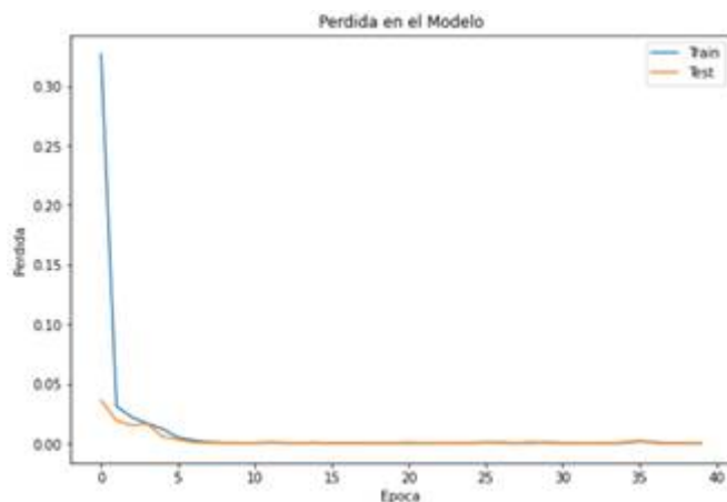
FIGURA 9. Tendencia Perdida del Modelo. Elaboración Propia
