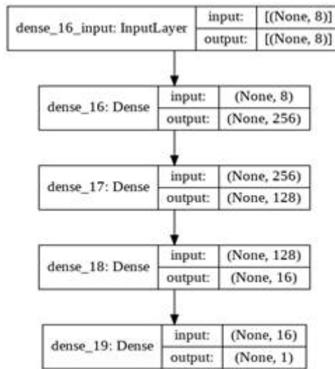
FIGURA 5. Modelo Secuencial de la RNA Elaboración Propia
