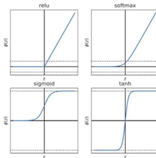
FIGURA 6. Funciones de Activación Elaboración Propia
