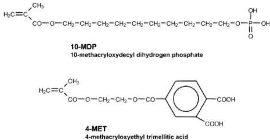
Figura 1. Estructura y grupos funcionales de la molécula de 10-MDP
