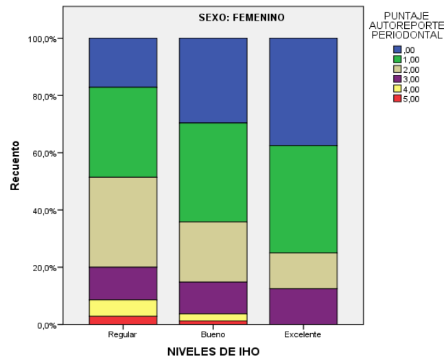
Gráfico 2. KENDALL 0.057
