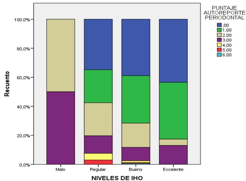
Gráfico 2. KENDALL 0.057
