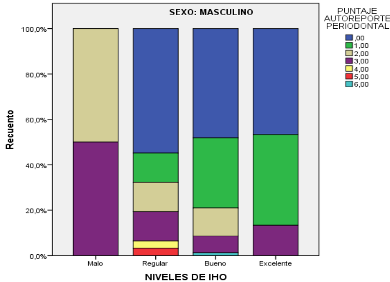
Gráfico 3 KENDALL 0.489
