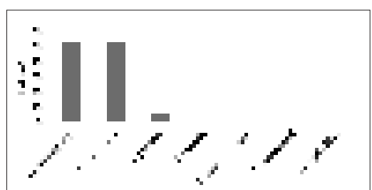
Figura 10. Densidad total de la Clase Thaliacea registrada en la ZII.
